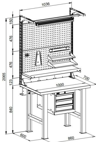
Верстак ДиКом ВС-100
