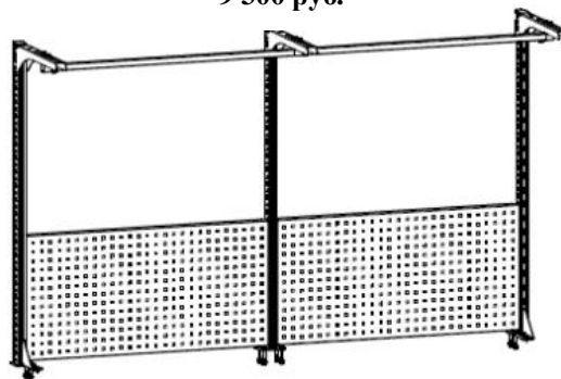
ДиКом ВС-200-Э3 Экран 8 390 руб.
