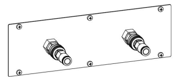
Вставка с 2 пневматическими БРС и цанговыми фитингами (шланг 10) 4 900 руб.
