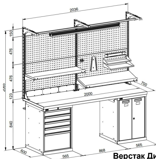
Верстак ДиКом ВС-150
