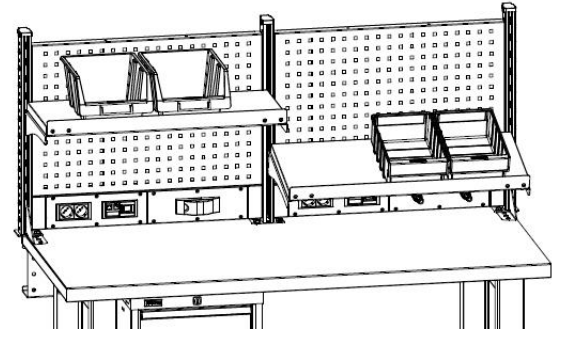
ВС Полки на экран можно установить прямо или под наклоном 15°
