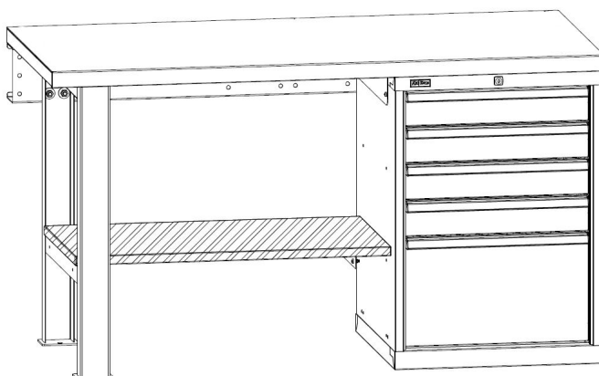
Пример использования Полки нижней с однотумбовым верстаком
