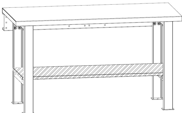
Пример использования Полки нижней с бестумбовым верстаком
